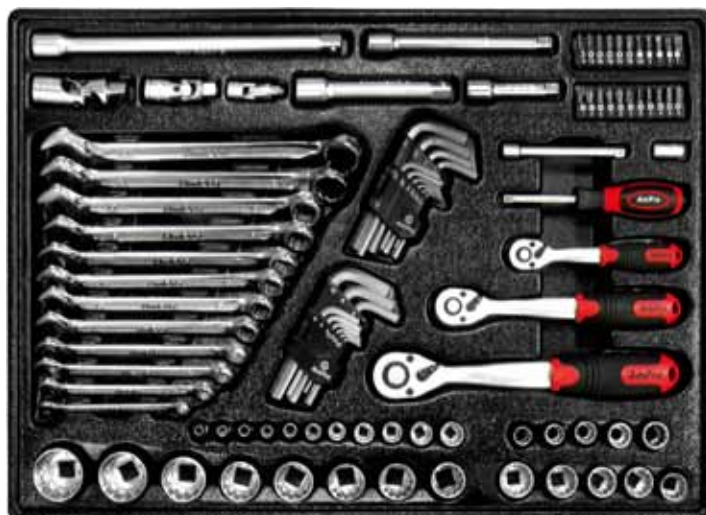
T45996 Набор универсальных головок и аксессуаров 1/4", 3/8", 1/2", 94 предмета*
